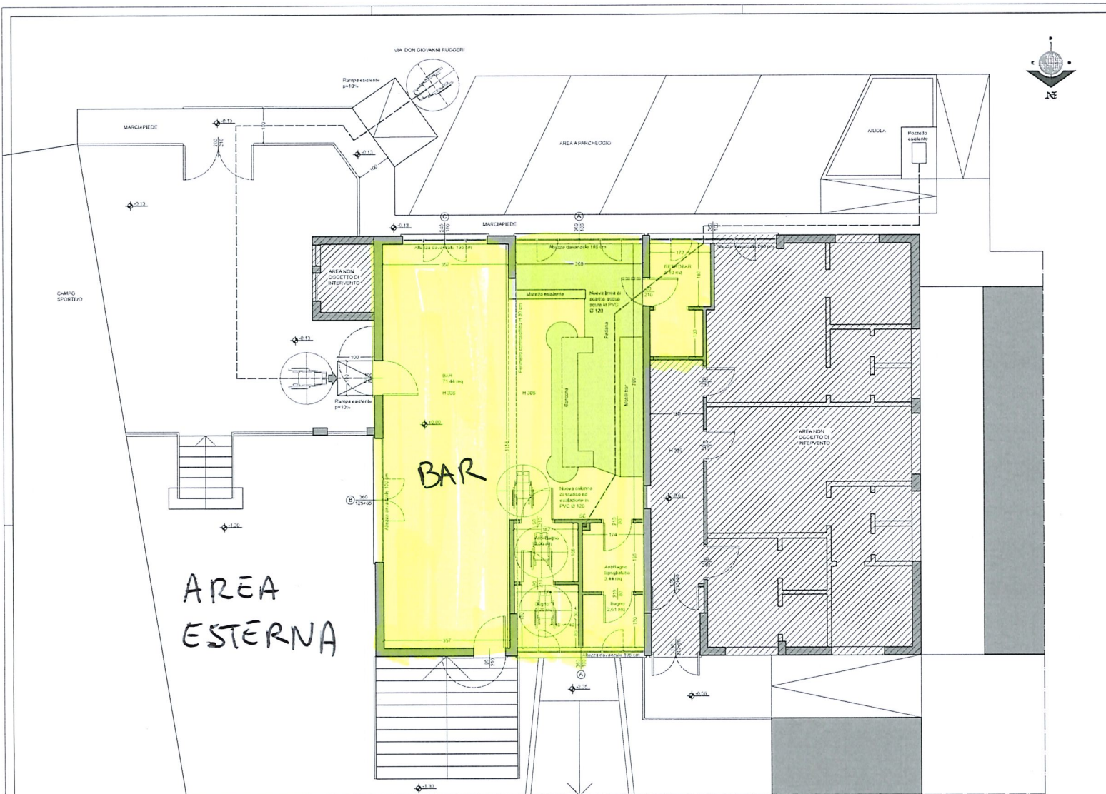
PIANTA DI PROGETTO - scala 1:50
