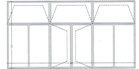
Ⓑ SERRAMENTO L.120 x H.110 x SOPRALUCE H.145
